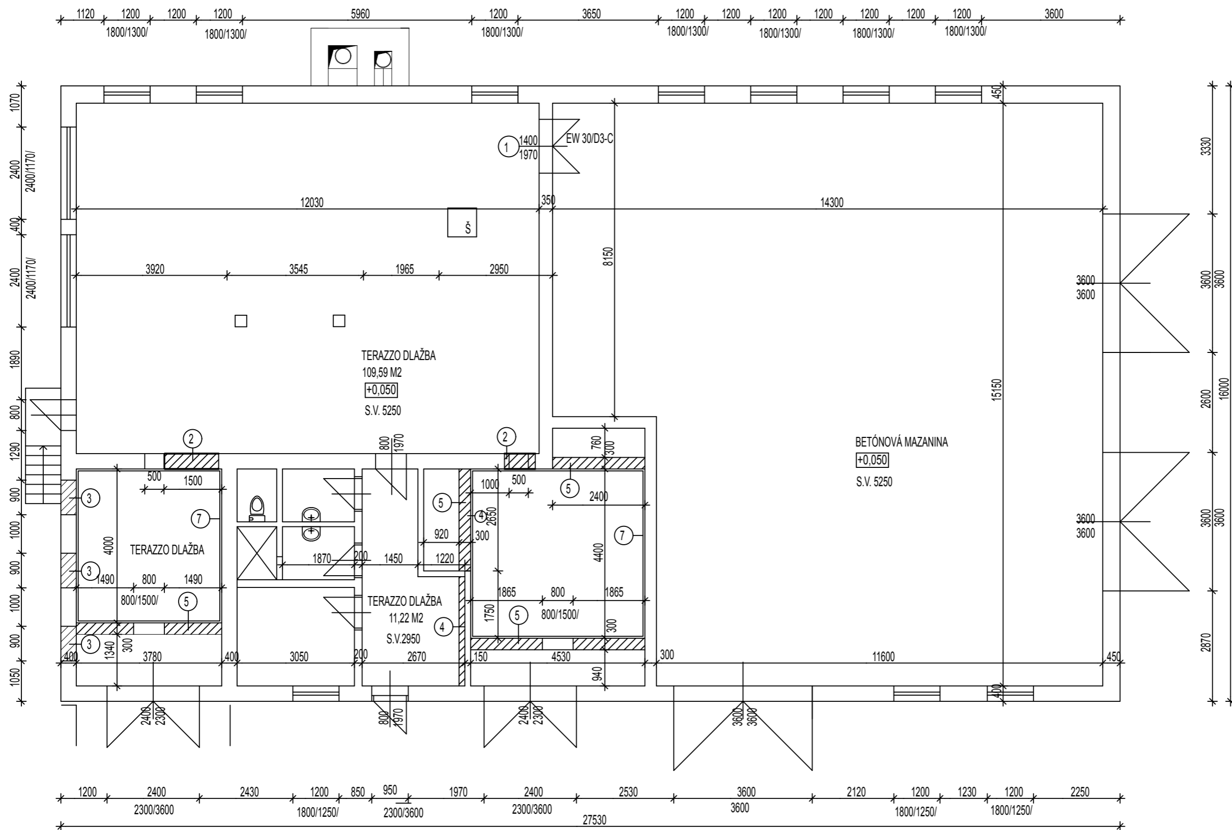
PÔDORYS KOTOLNE OÚ /M=1:100/ - nový stav
